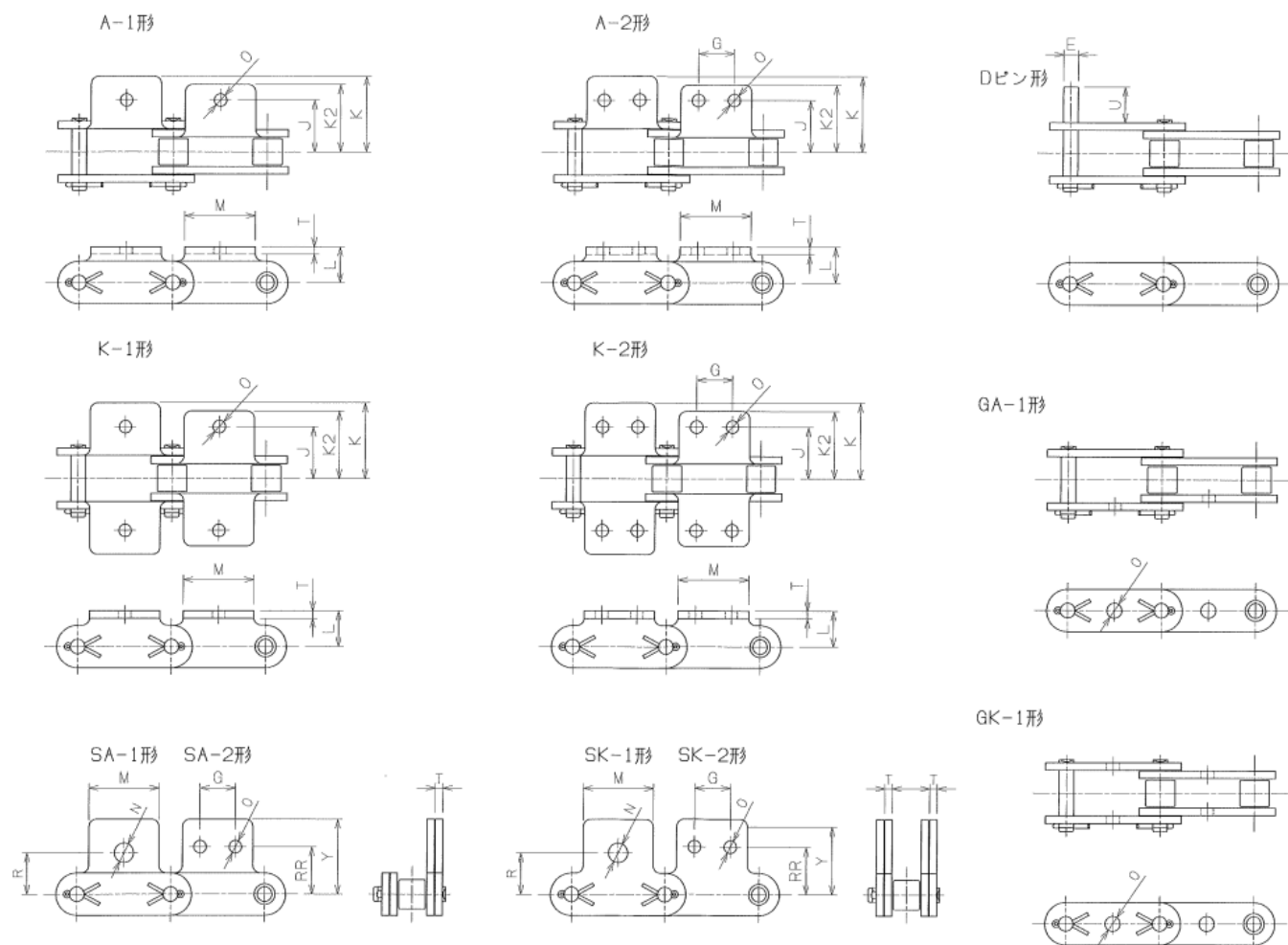
●ダブルピッチチェーン・アタッチメント寸法（S・Rローラ形）
